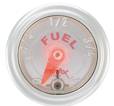
11256 - Füllstandsanzeiger kpl. für DT-Mobil Easy Pick-up 210 l
