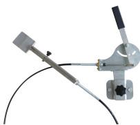
10208 - Fernbedienung mit Bowdenzug 2 m für Streuwagen SW 200 und SW 300
