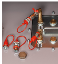
11506 - Entnahmeleitung für Generatortank kpl. für PRO ST Basic, 1x Vor. 1x Rücklauf
